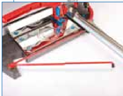
Braccio estensibile per grandi formati Extension arm for supporting big tiles
